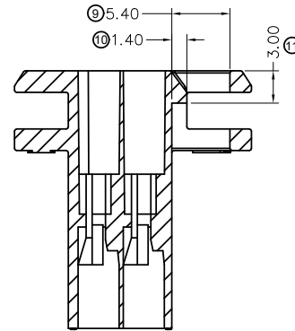
A-A SCALE 1:1
