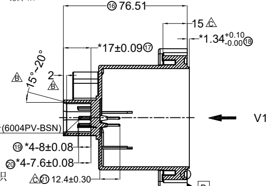
剖视图 B-B 比例 1:1
